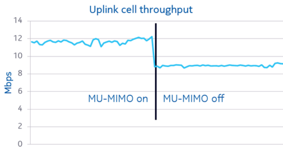
Рисунок 13. Увеличение пропускной способности восходящего канала на 40% при использовании многопользовательского MIMO
