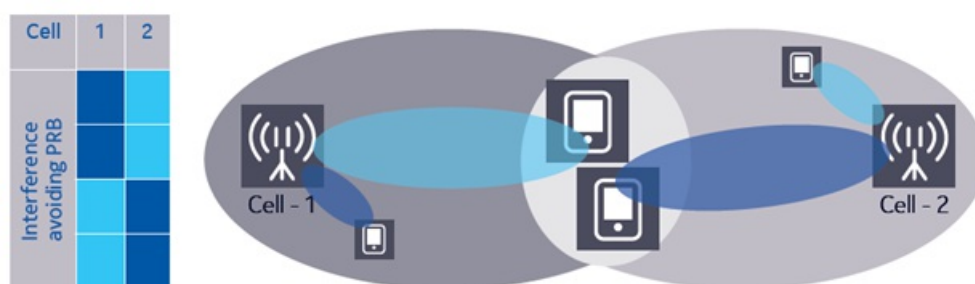
Рисунок 12 – Intelligent Beamforming для предотвращения межсотовых помех
