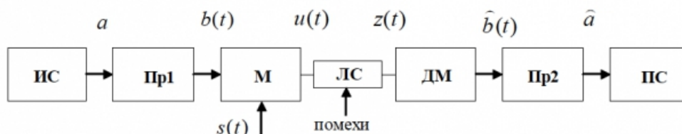
Рис. 1.2. Упрощённая структура системы связи
