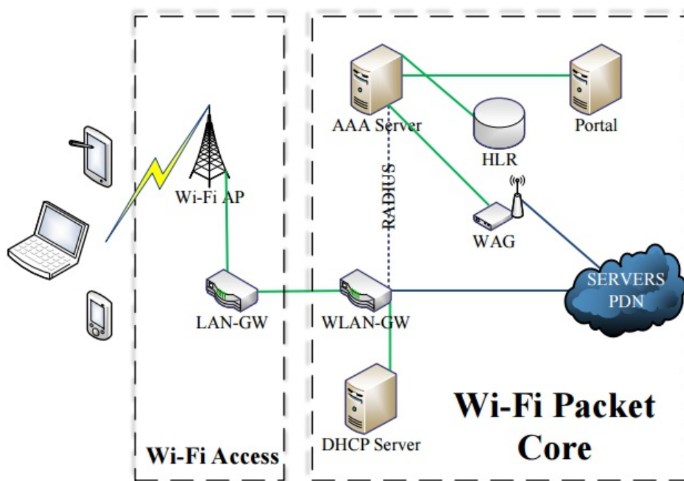
Рисунок 2 – Архитектура сети Wi-Fi
