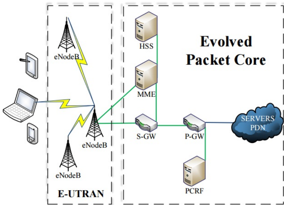
Рисунок 1 – Архитектура сети LTE
