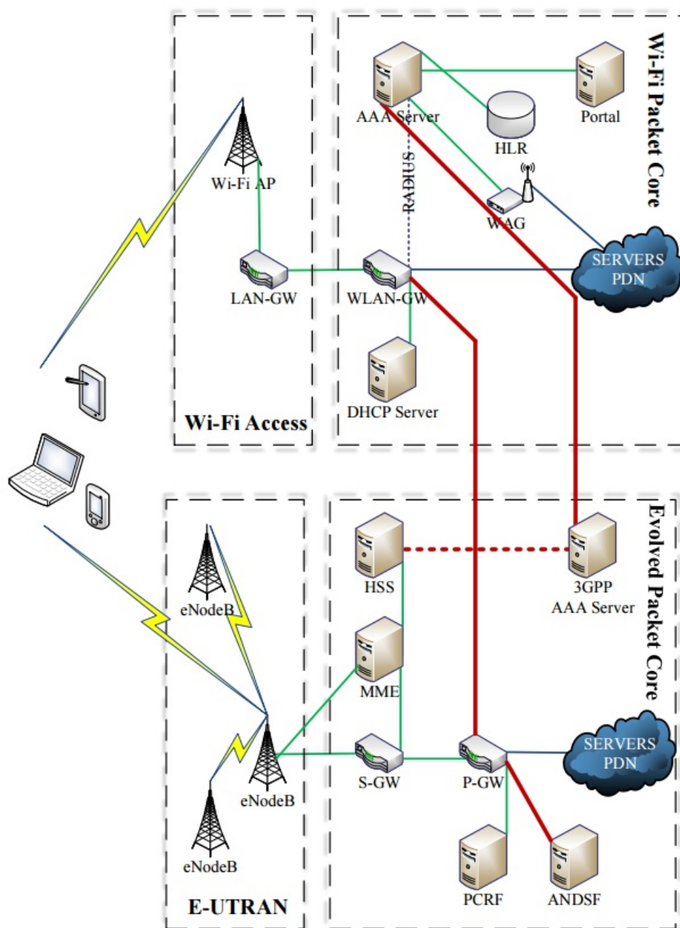
Рисунок 3 – Архитектура гибридной LTE-Wi-Fi сети
