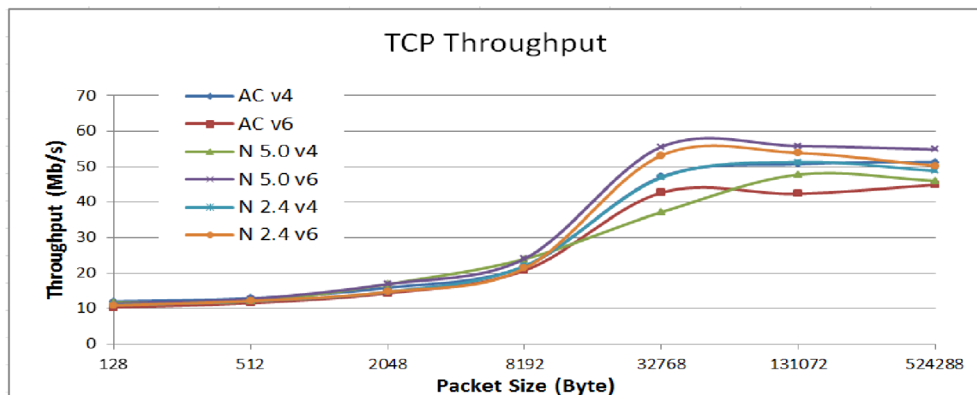
Рисунок 4 – Пропускная способность TCP трафика
