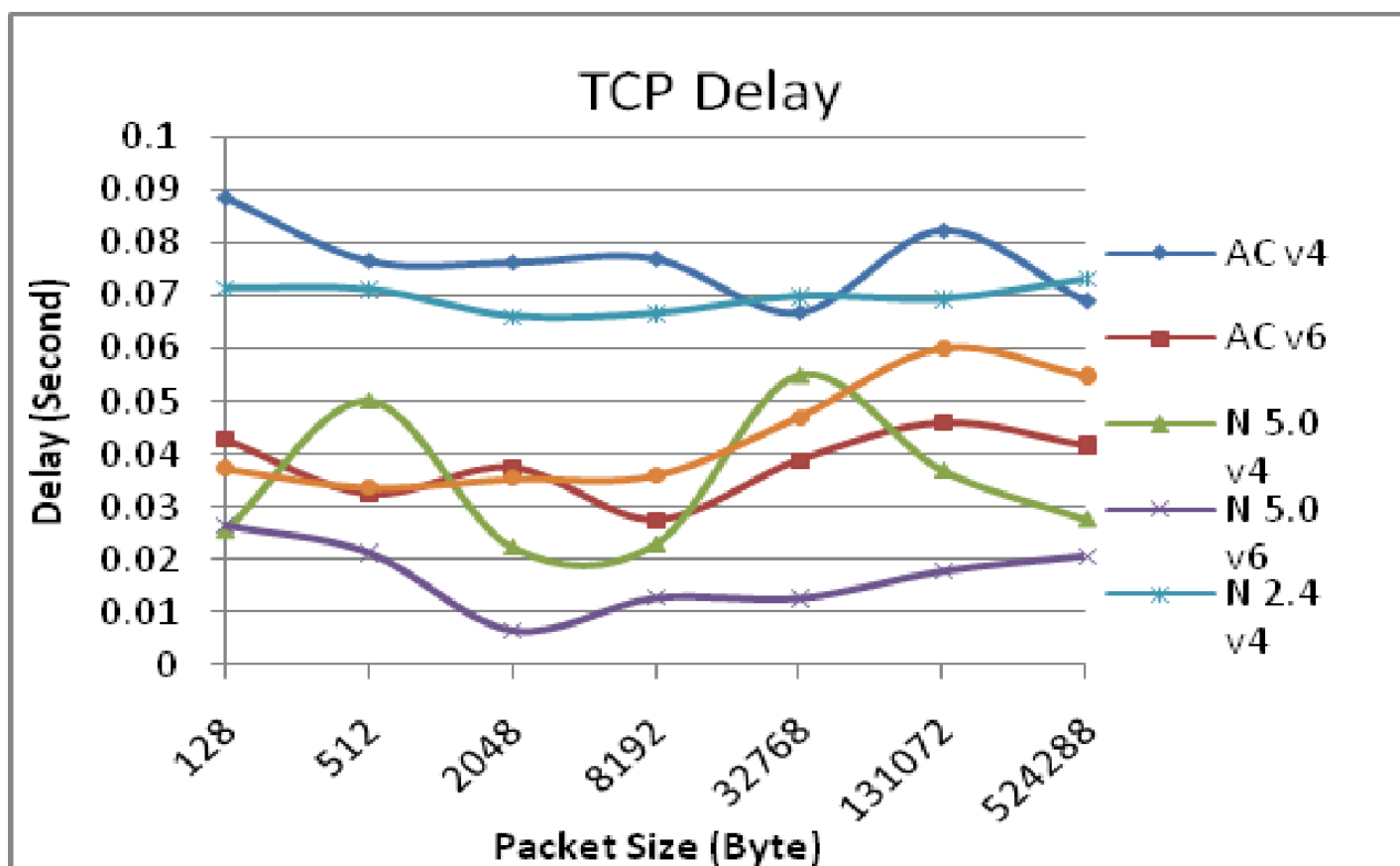
Рисунок 7 – Задержка TCP трафика
