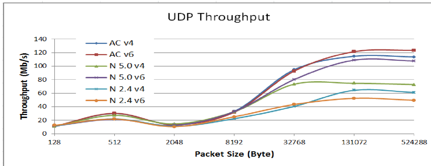
Рисунок 3 – Пропускная способность UDP-трафика
