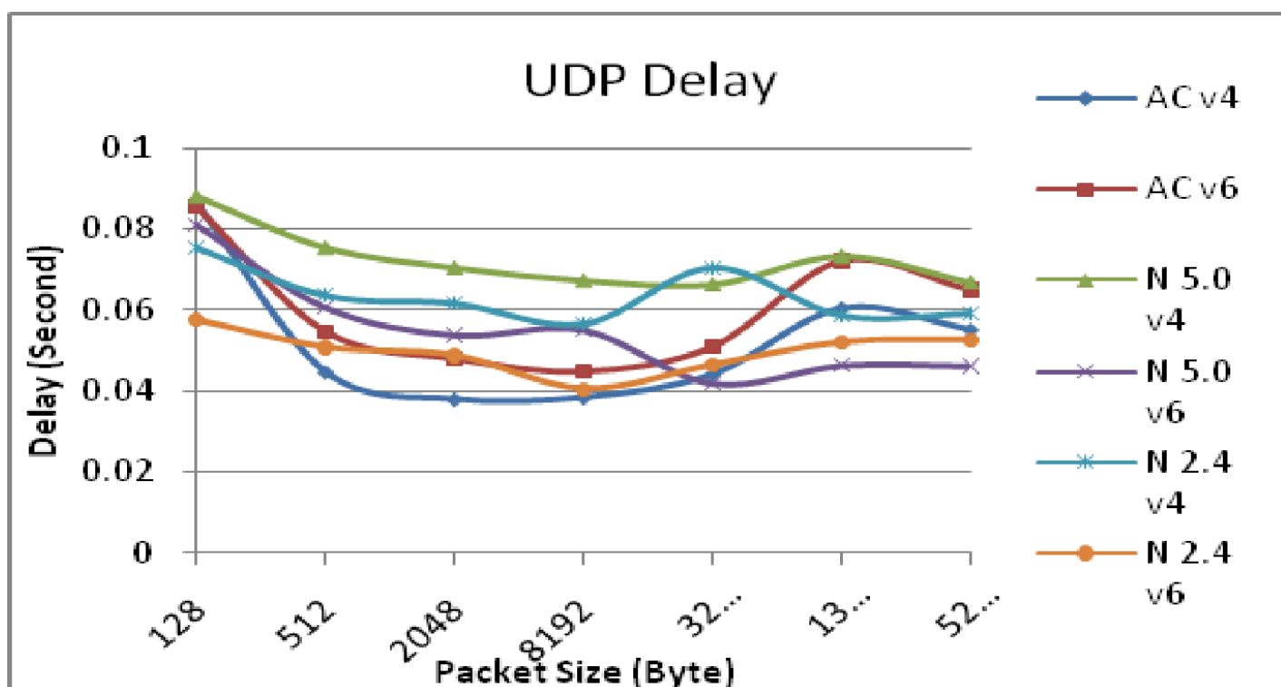
Рисунок 8 – Задержка UDP трафика
