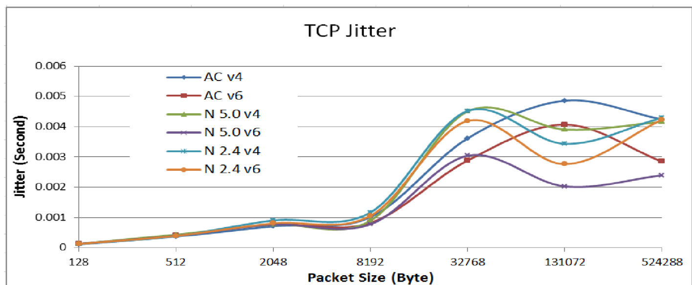
Рисунок 5 – Джиттер TCP трафика
