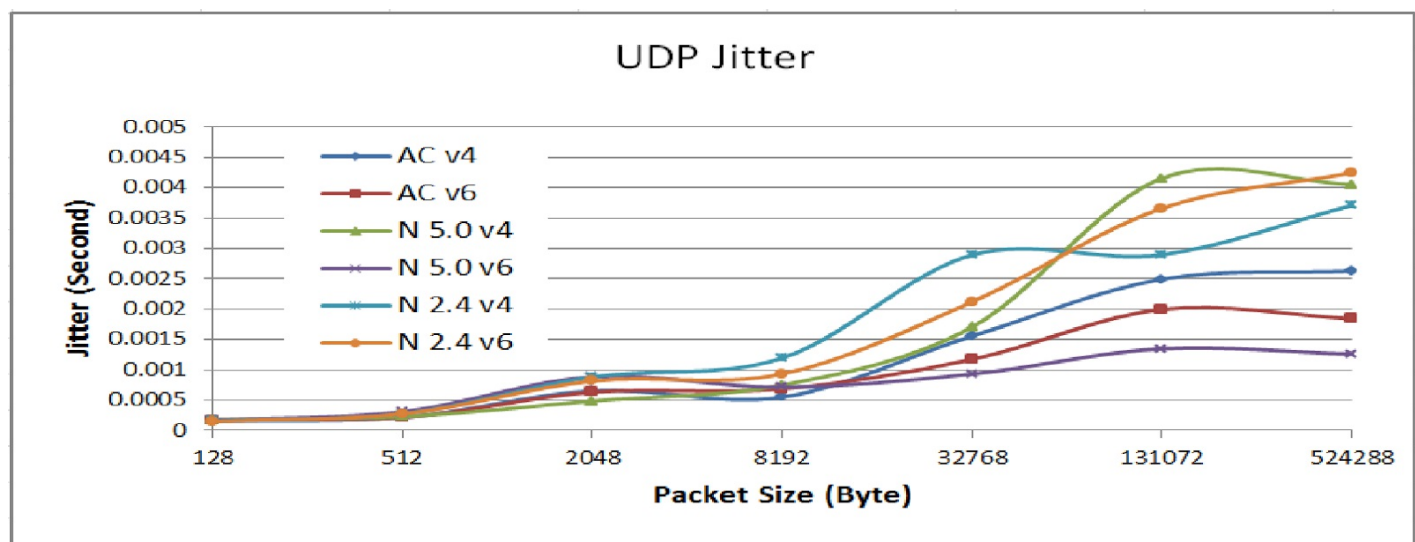
Рисунок 6 – Джиттер UDP – трафика
