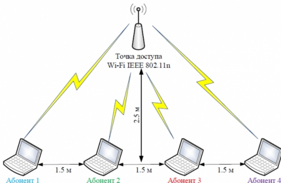
Рисунок 2 – Подключение абонентов к точке доступа
