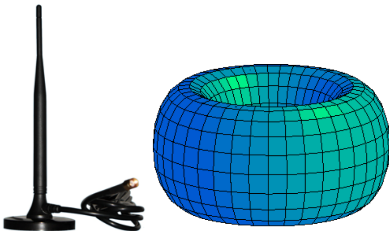
Рисунок 1 – Внешний вид и диаграмма направленности Omni-антенны
