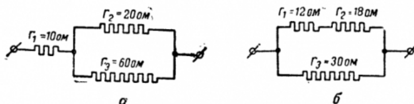
Рис. 15. Смешанное соединение сопротивлений: а и б — случаи соединения сопротивлений
