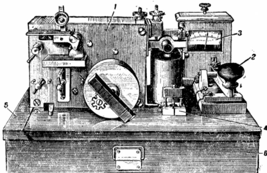
Рис. 118. Аппарат Морзе военного образца 1910 г.: 1 — пишущий приёмник; 2 — ключ-передатчик; 3 — гальваноскоп; 4 — переключатель тока; 5 — цоколь; 6 — tambour для ленты
