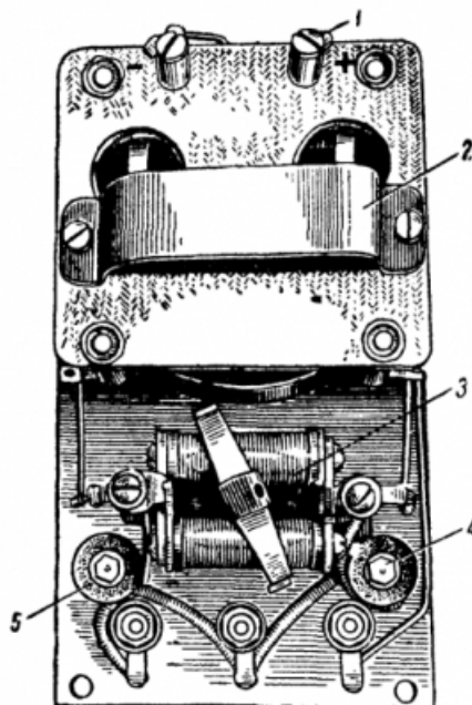
Рис. 102б. Вид на панель омметра типа ОДО-1 снизу: 1 — контактные колонки; 2 — скобка; 3 — рео- стат; 4 и 5 — катушки сопротивления
