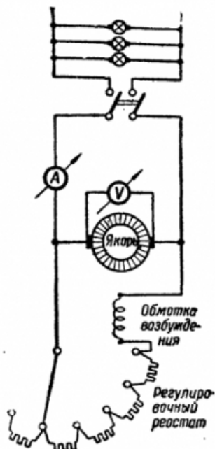
Рис. 66. Схема включения динамомашины с параллельным возбуждением
