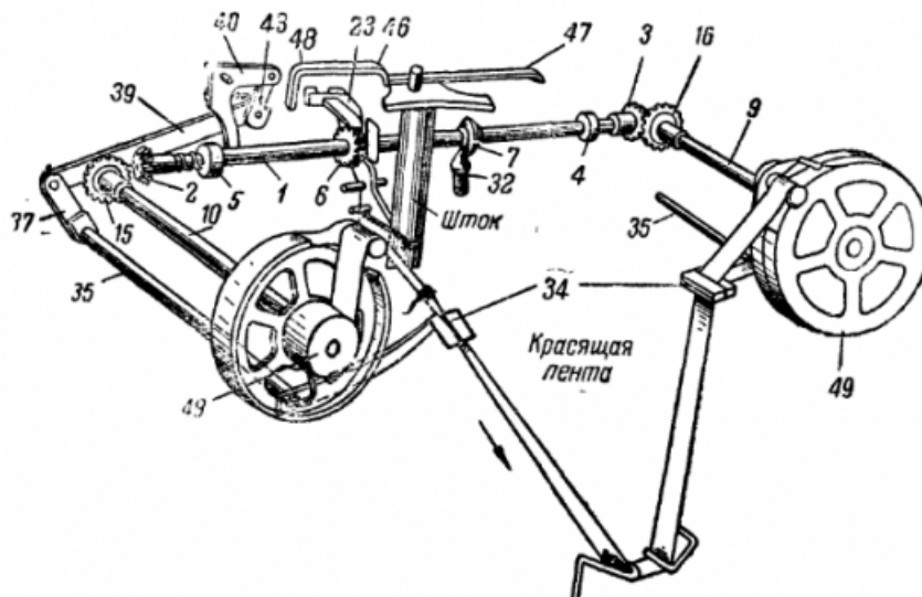
Рис. 200. Взаимодействие деталей механизма продвижения красящей ленты:
