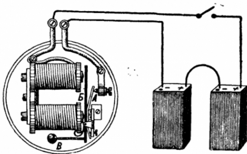
Рис. 47. Электромагнит звонка постоянного тока (неполяризованный электромагнит)
