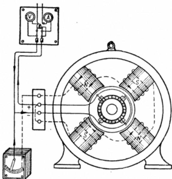
Рис. 65. Динамомашинa с параллельным возбуждением
