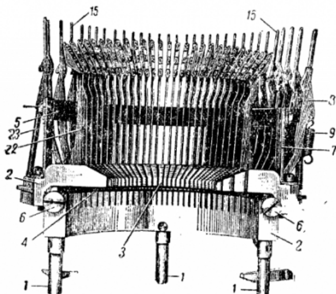
Рис. 192. Сегмент с типовыми рычагами:
