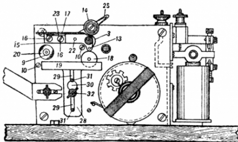
Рис. 129а. Лентопротяжное приспособление (вид спереди):
