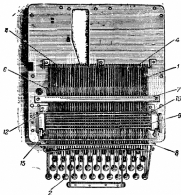
Рис. 169г. Вид на детали клавиатуры снизу:
