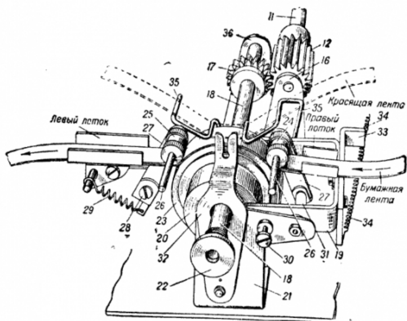
Рис. 195а. Лентопротяжная каретка механизма продвижения бумажной ленты аппаратов новых выпусков:
