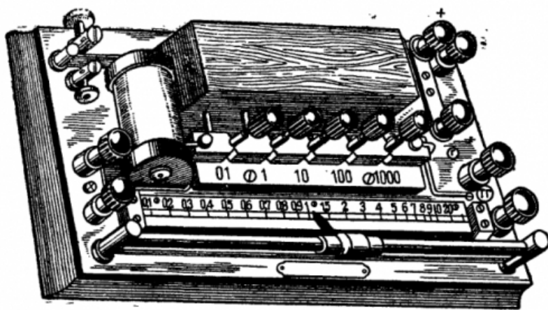
Рис. 105. Мост Кольрауша
