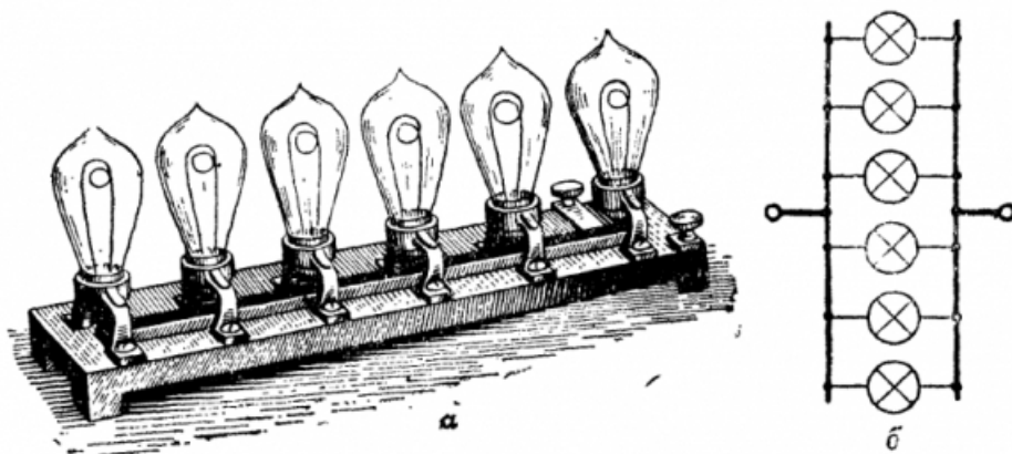
Рис. 19. Ламповый реостат: а — внешний вид; б — схематическое изображение
