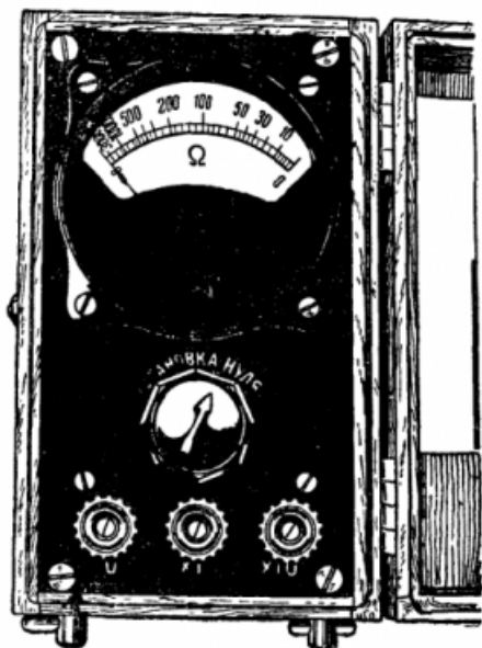
Рис. 102а. Омметр типа ОДО-1 (вид сверху)
