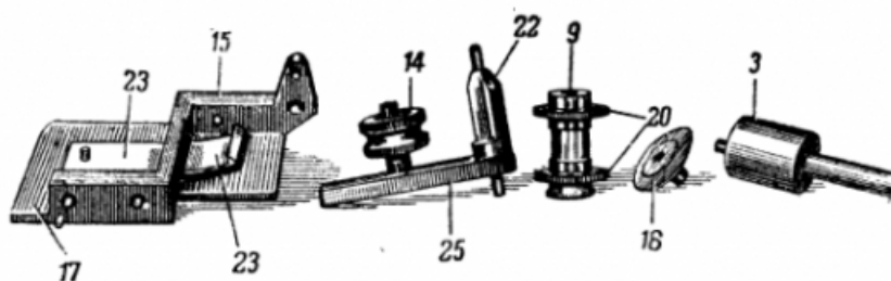
Рис. 129б. Части лентопротяжного приспособления:
