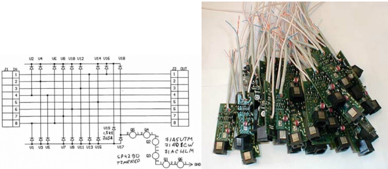
Схема оригинальной защиты APC (слева) и ее самодельные аналоги (справа)
