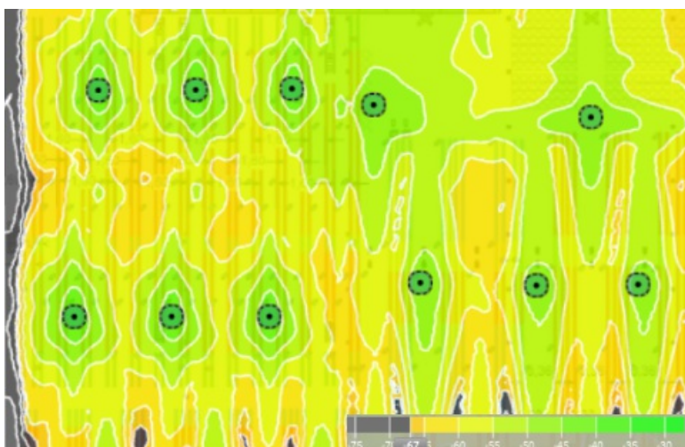
Рис. 3. Пример расположения точек доступа и моделирование уровня сигнала в 5 ГГц.
