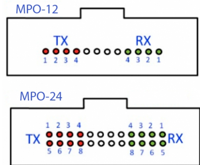
Рисунок 2. Схема распределения каналов для MPO
