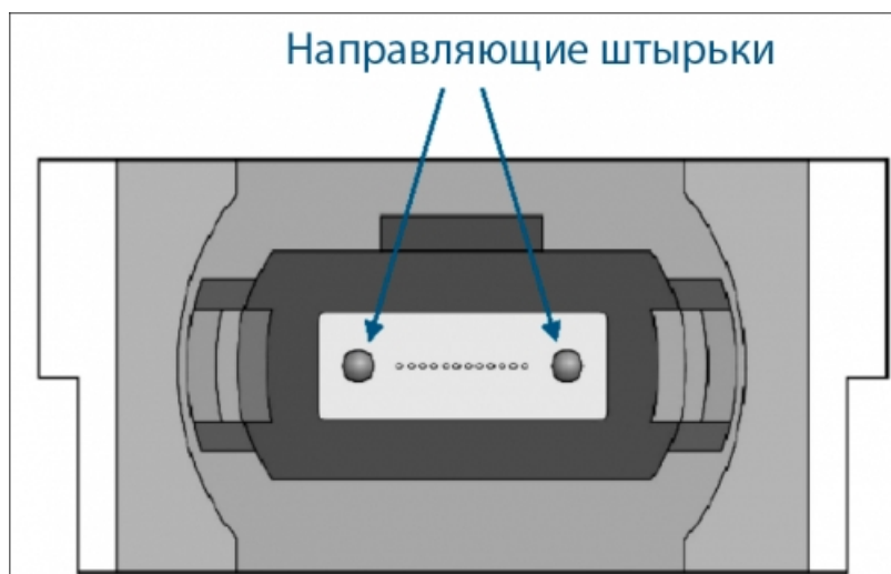
Рисунок 1. Разъем MPO оптического модуля 40/100G
