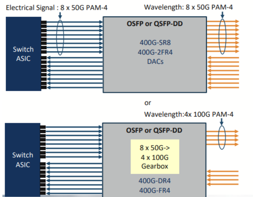
Рисунок 4. Структурная схема устройства модуля
