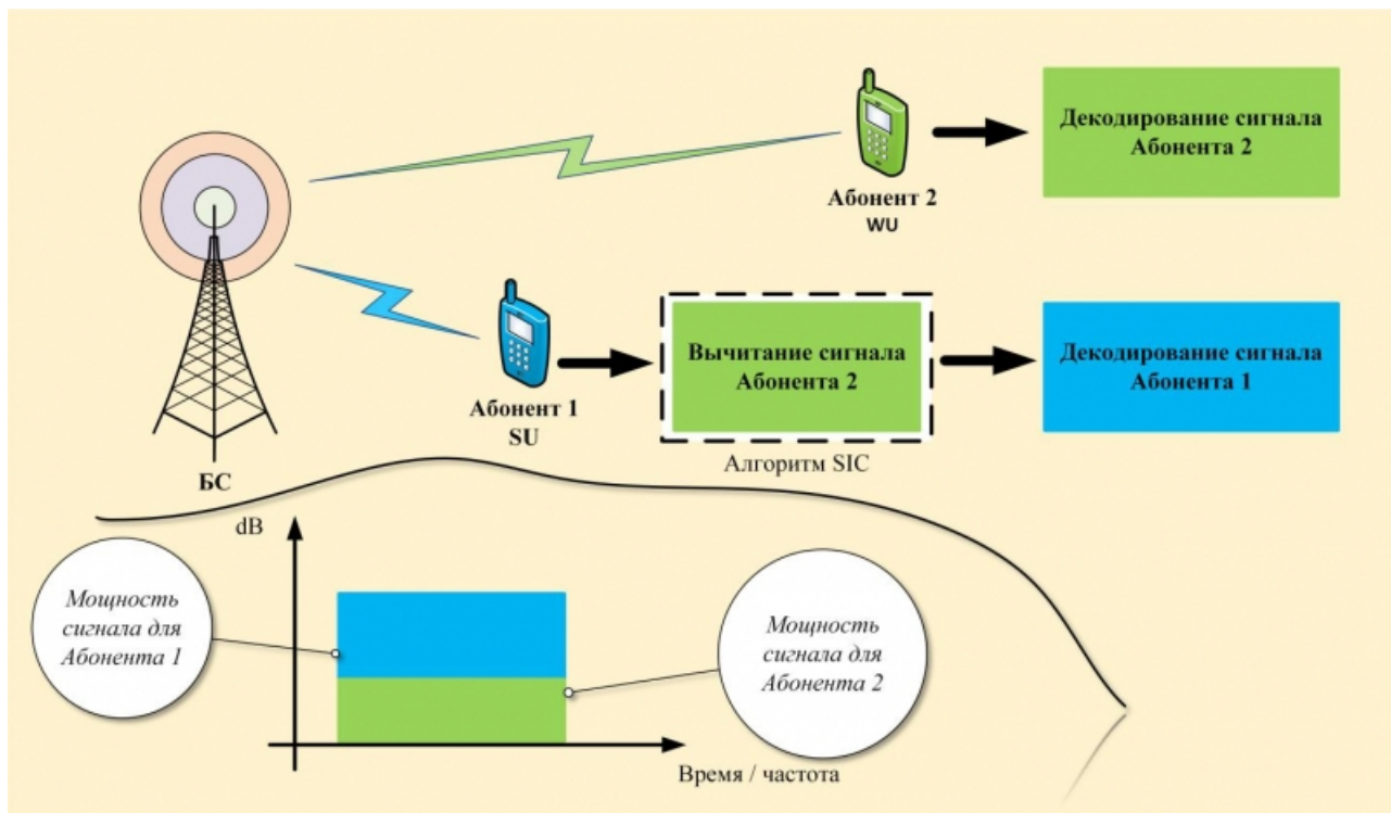
Рисунок 1 - Принцип работы NOMA в нисходящем канале
