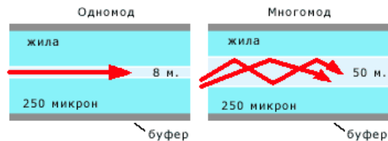
Отличия одномодового и многомодового волокна.
