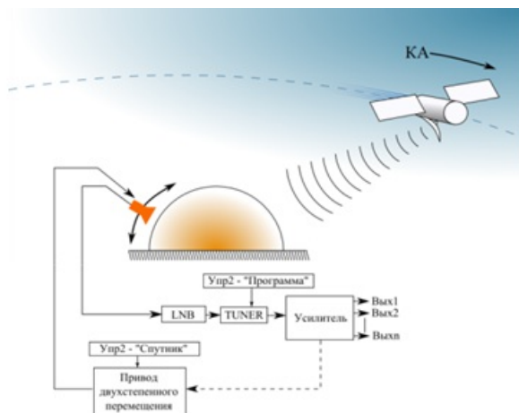
Рис. 1.7 – ЛЛ на движущемся объекте
