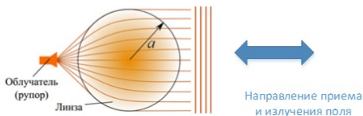
Рис. 3 – Схема прохождения лучей через линзу Люнеберга
