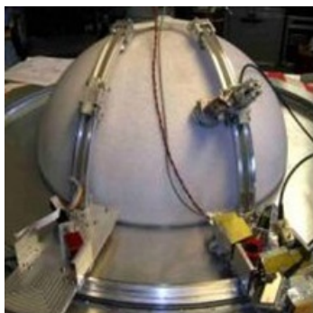
Рис. 9 – Устройство перемещения первичного облучателя ЛЛ
