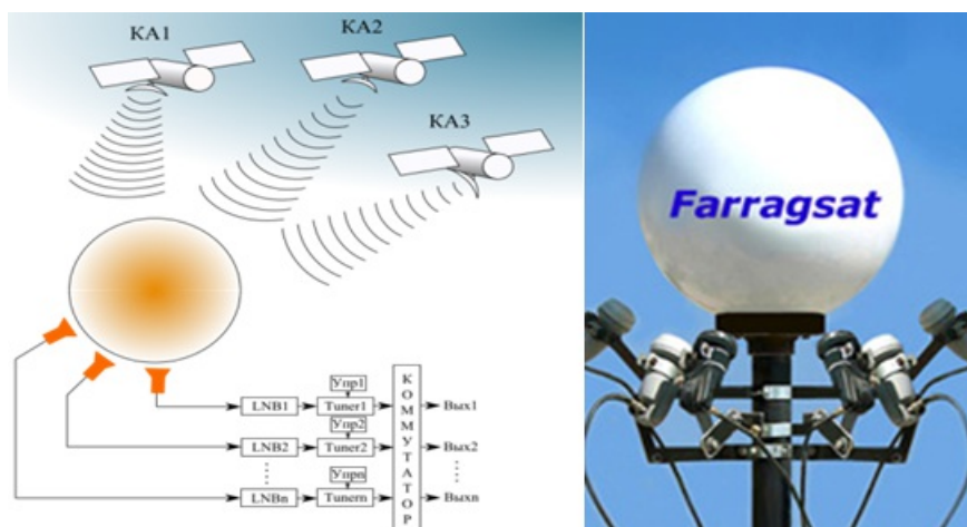
Рис. 7 – Многоканальный терминал спутниковой связи с ЛЛ
