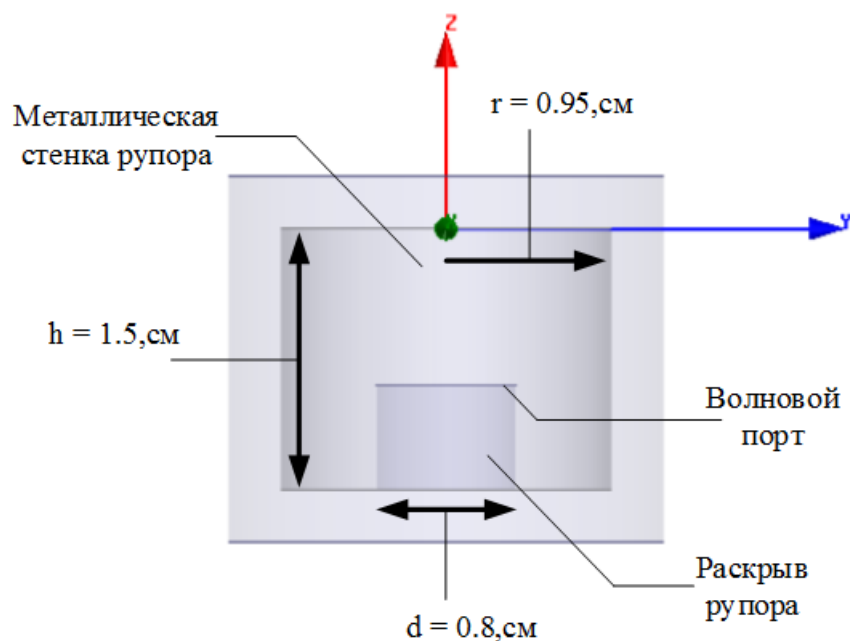
Рис. 12 – Модель первичного облучателя ЛЛ в Ansys
