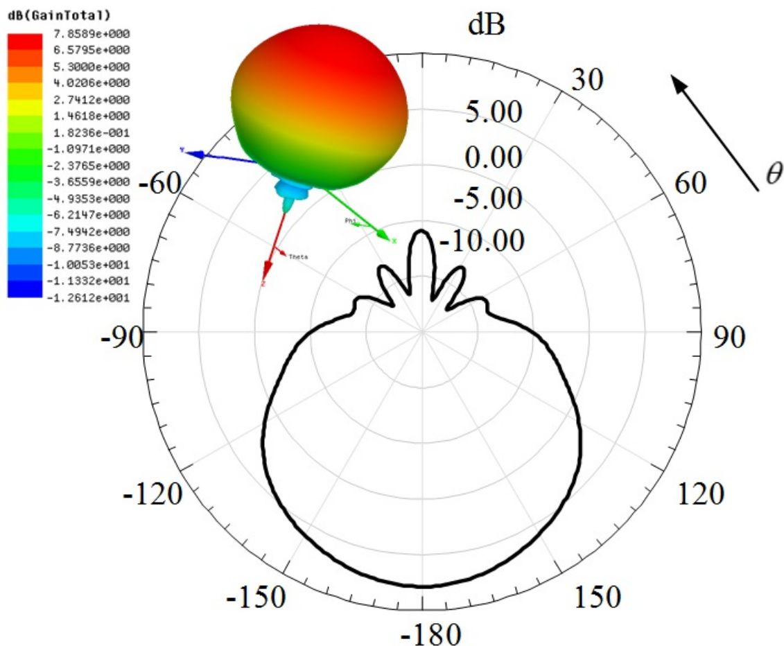
Рис. 12 – Диаграмма направленности рупора
