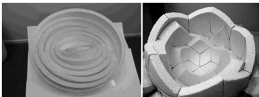
Рис. 4 – Конструктивная реализация многослойной линзы
