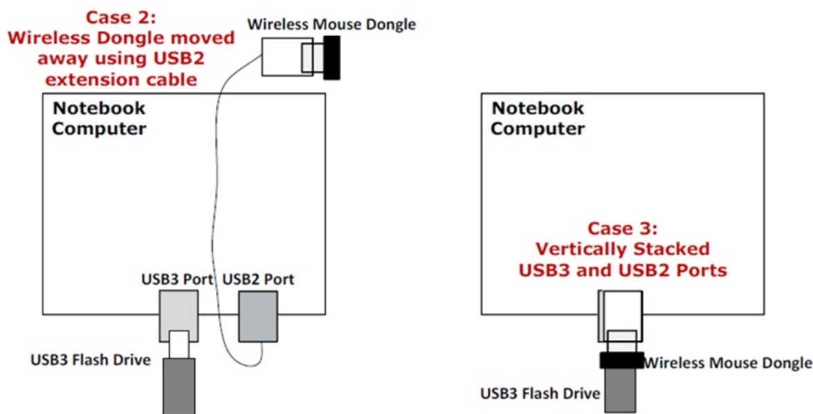
Рисунок 16 – Влияние расположения USB-устройства на антенну радиоприемника
