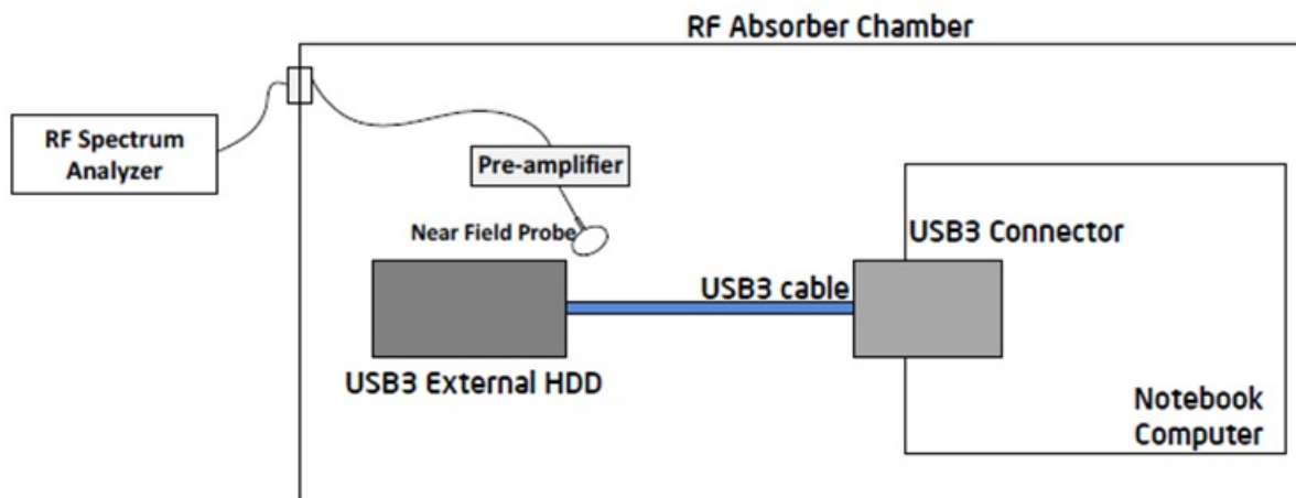
Рисунок 4 – Экспериментальная установка для измерения шума от внешнего USB 3.0 жесткого диска
