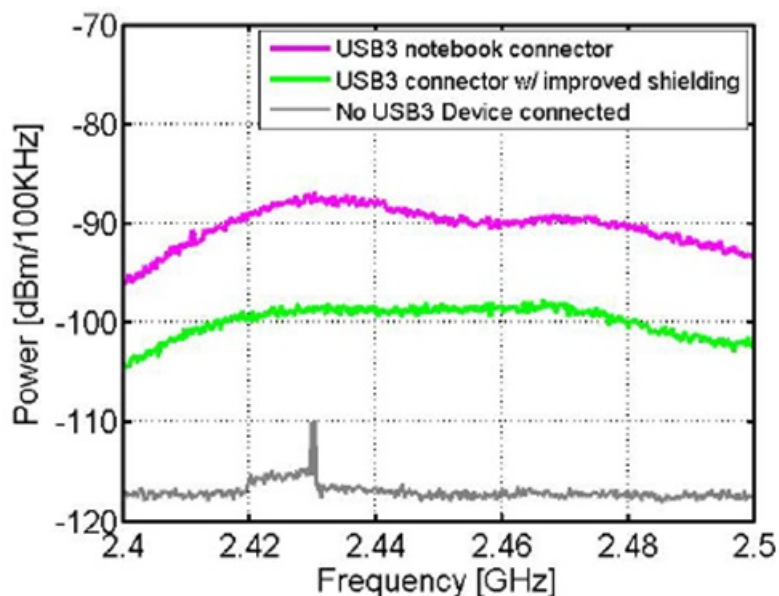
Рисунок 14 – Уровень шумов от USB-разъема с улучшенным экранированием
