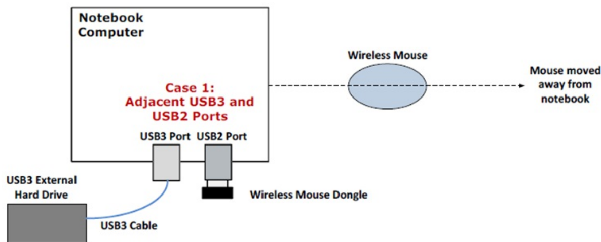
Рисунок 6 – Установка для измерения производительности беспроводной сети при наличии USB 3.0-устройства
