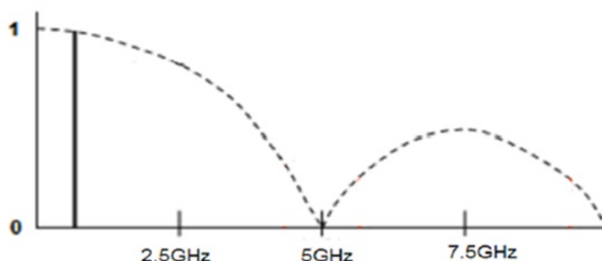
Рисунок 1 – Спектр передаваемых данных по интерфейсу USB 3.0, описанный sinc-функцией
