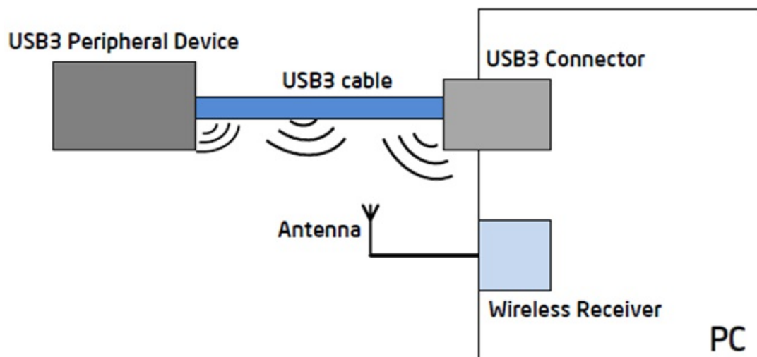
Рисунок 3 – Каналы излучения интерфейса USB 3.0
