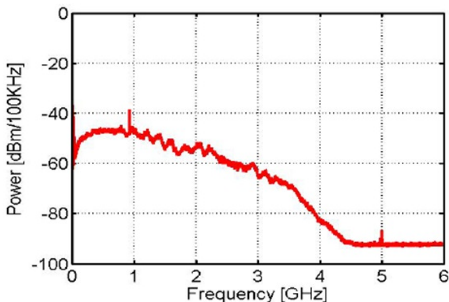
Рисунок 2 – Экспериментально измеренный спектр передаваемых данных по USB 3.0
