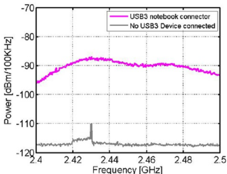
Рисунок 13 – Вклад уровня шумов от разъема USB 3.0
