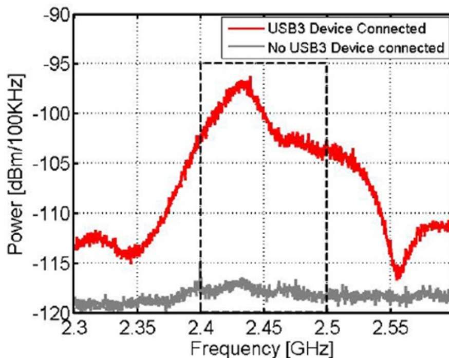
Рисунок 5 – Результаты измерения шума от внешнего USB 3.0 жесткого диска
