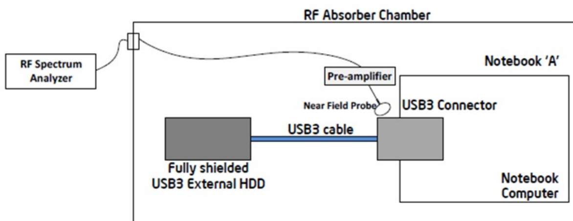
Рисунок 12 – Схема установки для измерения шума от USB-разъема
