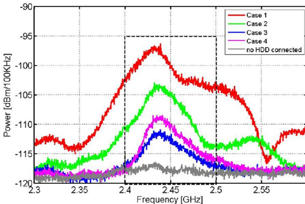
Рисунок 11 – Влияние экранирования USB 3.0-устройства на уровень сигнала
