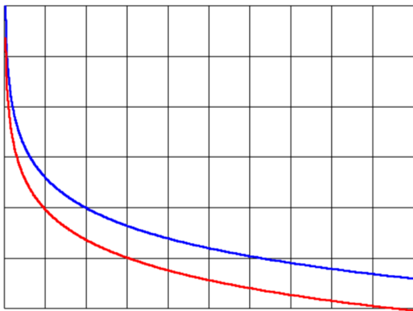
Рисунок 1 – затухание сигнала Wi-Fi с увеличением расстояний
