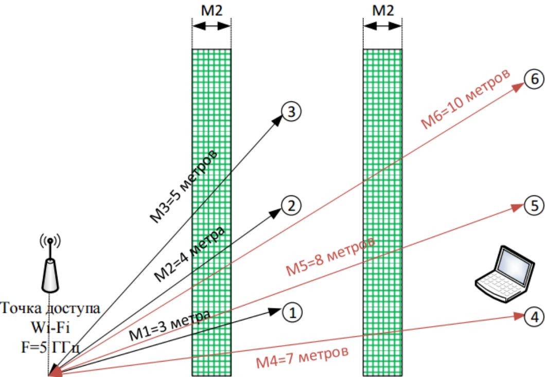
Рисунок 3 – Расстояния от точки доступа до точки измерения
