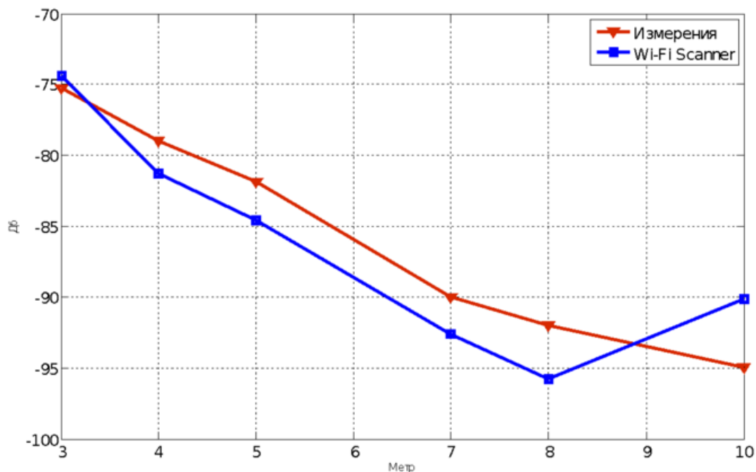
Рисунок 4 – Результаты расчетов и измерений
