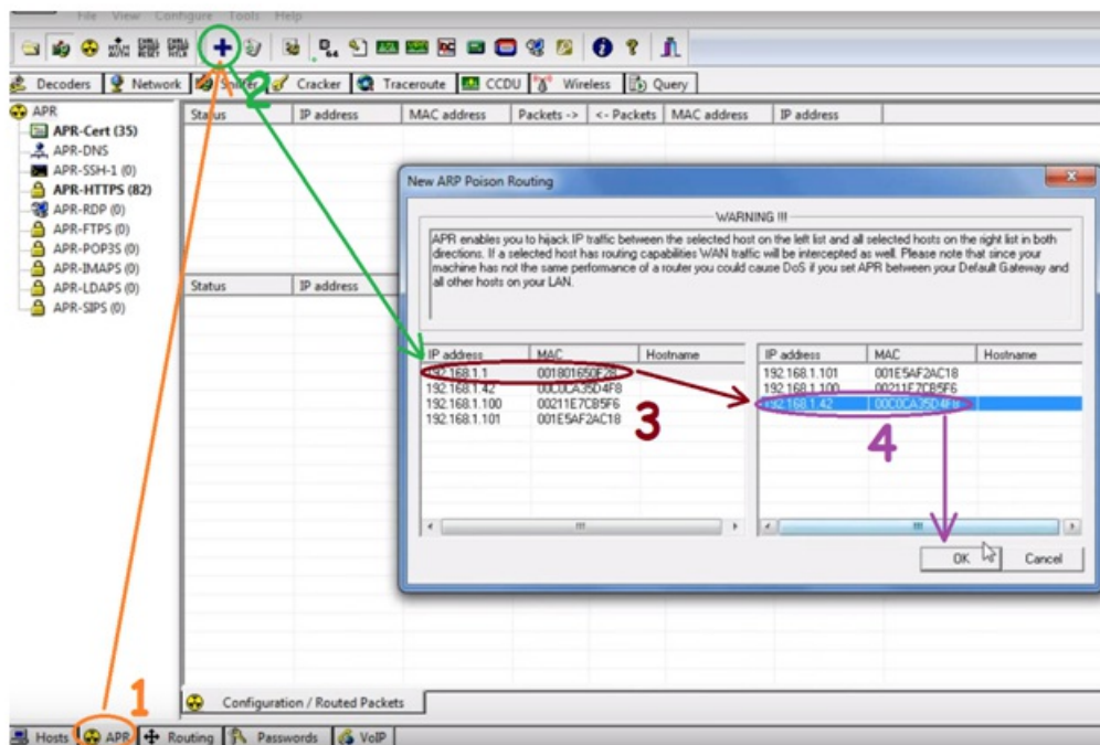
Рисунок 10 – Модификация протокола ARP
