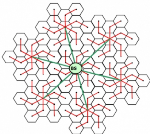
Рисунок 3. E – Конфигурация сети multi-tier 1:7:91; 3 хопа
