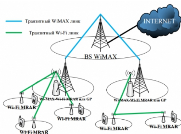
Рисунок 1 – Архитектура сети multi-tier WiMAX-Wi-Fi
