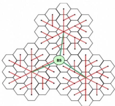
Рисунок 3. F – Конфигурация сети multi-tier 1:3:57; 3 хопа
