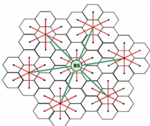
Рисунок 3. С – Конфигурация сети multi-tier 1:7:49; 2 хопа
