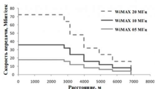
Рисунок 5 – Зависимость скорости передачи данных WiMAX транзитного линка от расстояния для каналов шириной 5, 10, и 20 МГц.
