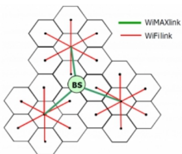
Рисунок 3. В – Конфигурация сети multi-tier 1:3:21; 2 хопа
