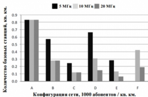
Рисунок 6 – Минимальное количество базовых станций для 1000 абонентов на кв. км.
