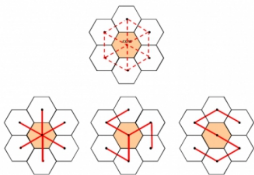
Рисунок 2 – Двухуровневая топология формирования сети (пример для семи ячеек в кластере)
