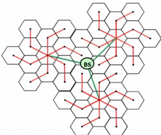
Рисунок 3. D – Конфигурация сети multi-tier 1:3:39; 3 хопа
