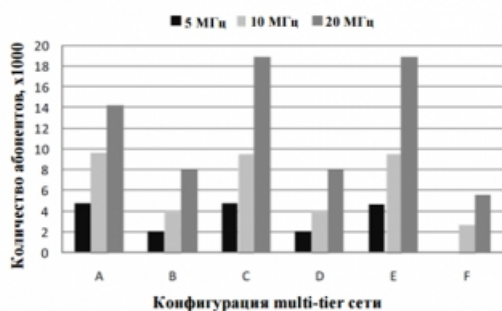
Рисунок 6 – Максимальное количество абонентов для multi-tier сетей (A-F)
