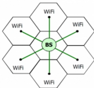
Рисунок 3. А – Конфигурация сети multi-tier 1:7:7; 1 хоп
