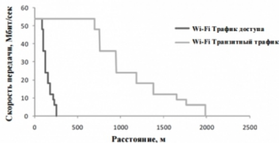
Рисунок 4 – Зависимость скорости передачи данных Wi-Fi от расстояния для линка доступа и транзитного линка
