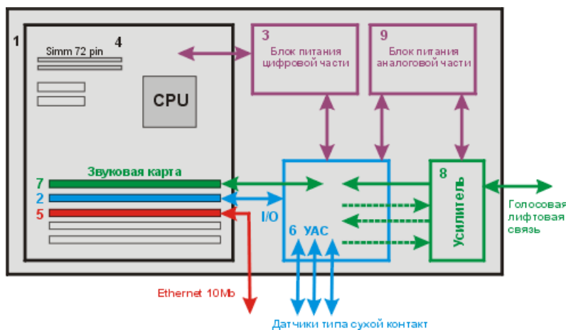
Схема установочного блока коммунального компьютера.
