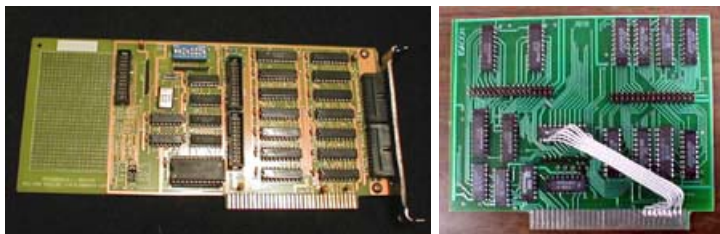
Слева показана плата PCL-720 rev. c4 digital I/O 64/64, послужившая прототипом.
