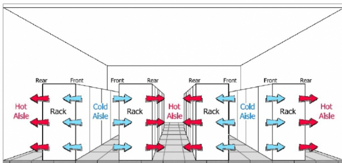
Чередование холодных и горячих коридоров
