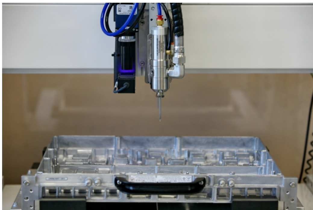
Процесс нанесения термогеля автоматизирован
