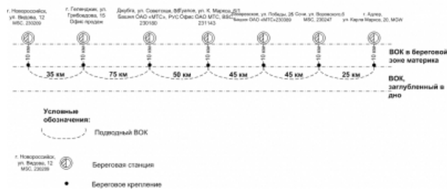
Схема организации линий связи планируемой Южной ВОЛП г.Новороссийск – г. Адлер
