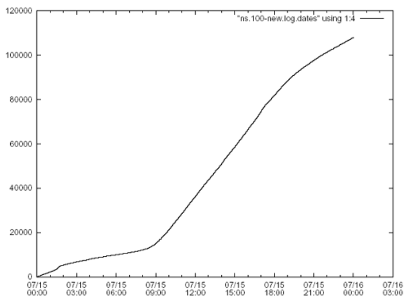
Рис. 2: Кумулятивное число новых dstip, история ограничена ста последними адресами, тот же лог.
