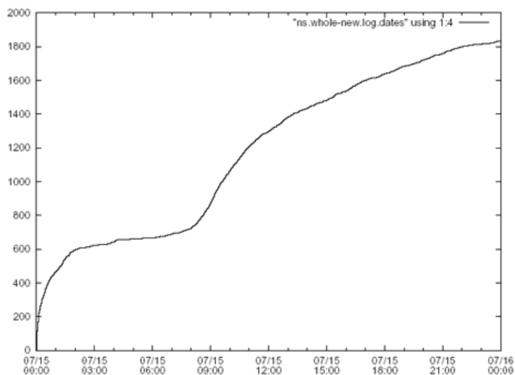
Figure 1: Кумулятивное число новых dstip, DNS сервер, 24-х часовой период
