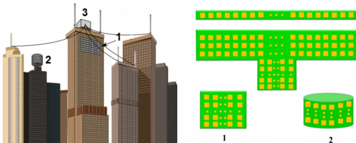
Рисунок 7 – Вид реализуемых геометрий M-MIMO (справа) и их возможное расположение в мегаполисе (слева)
