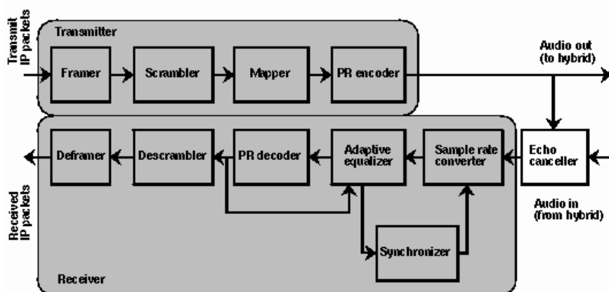
Схема работы блоков AuDSL.
