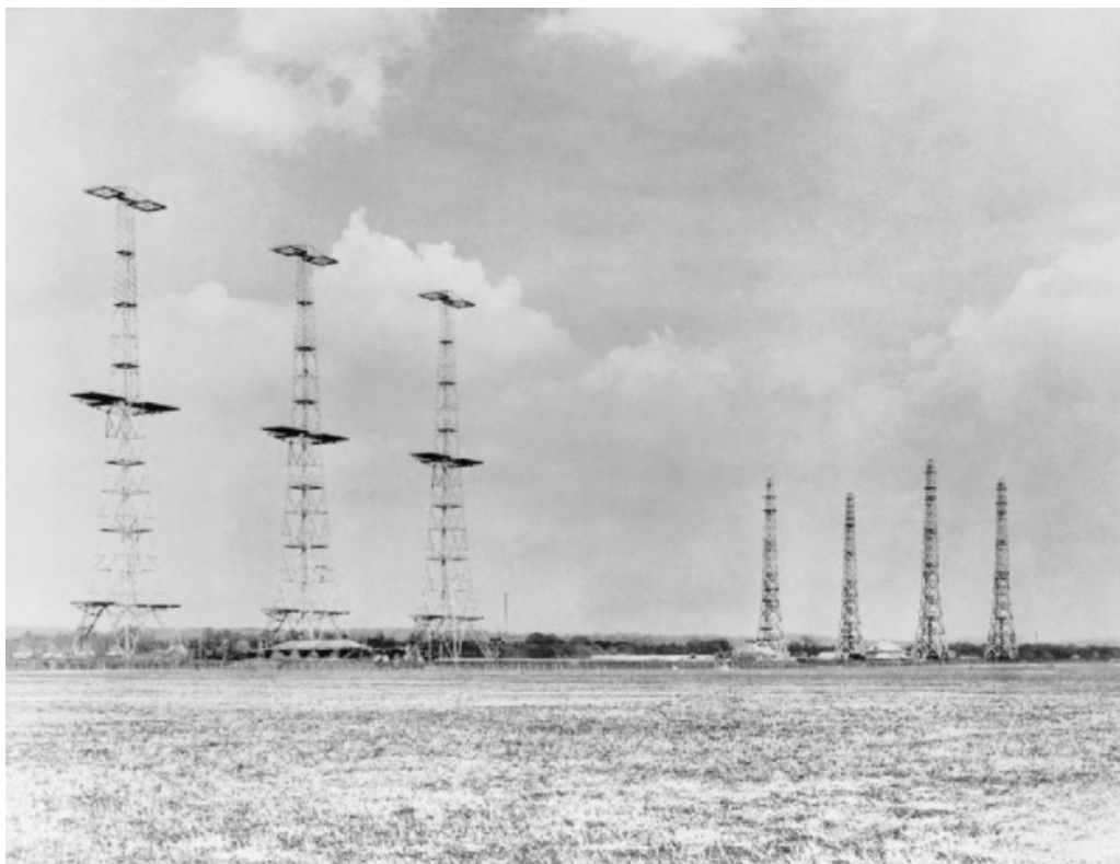
Радарные башни системы Chain Home.
