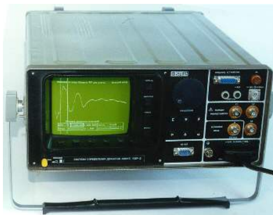
Изобретение совсем не ново. Подобные приборы используются с незапамятных времен. Так выглядит, например, рефлектометр К6Р5 советского производства.
