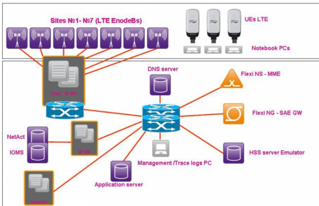
Схема тестовой сети LTE от компании Tele2 в Омске
