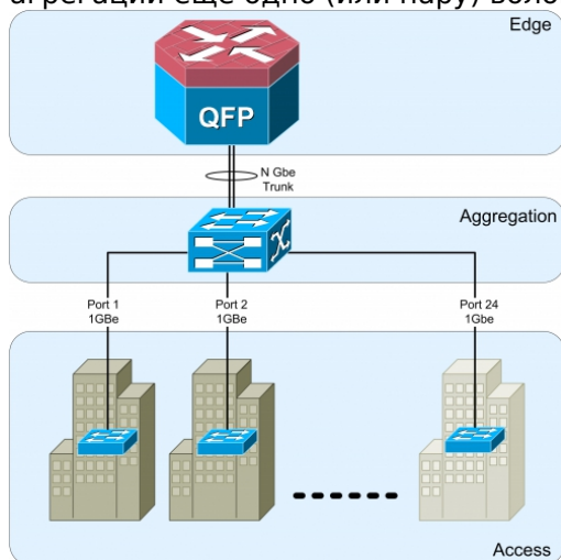
Объединение портов (транк)
