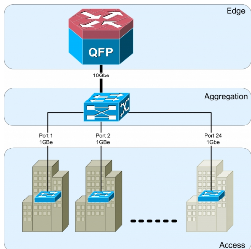
Узел агрегации с использованием 10G
