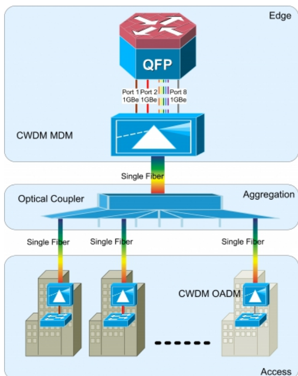
Схема с использованием CWDM
