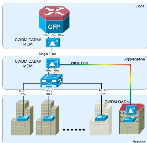
Совместное использование CWDM и коммутатора
