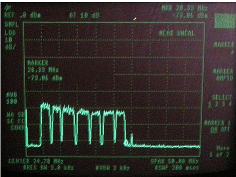
Рис. 2 Спектр Mode6
