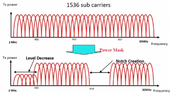
Рис 1. Спектр PLC сигнала
